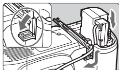
Orifice pour cordon du coupleur CC
